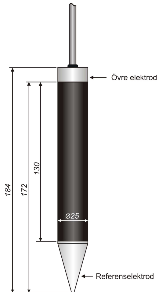
Bild 5. Måttitning av givaren OMS
