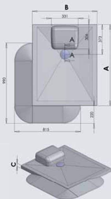
Traymatic Intern finns i 3 storlekar A×B×C: 1000×800×50 mm A×B×C: 900×900×50 mm A×B×C: 1200×800×50 mm
