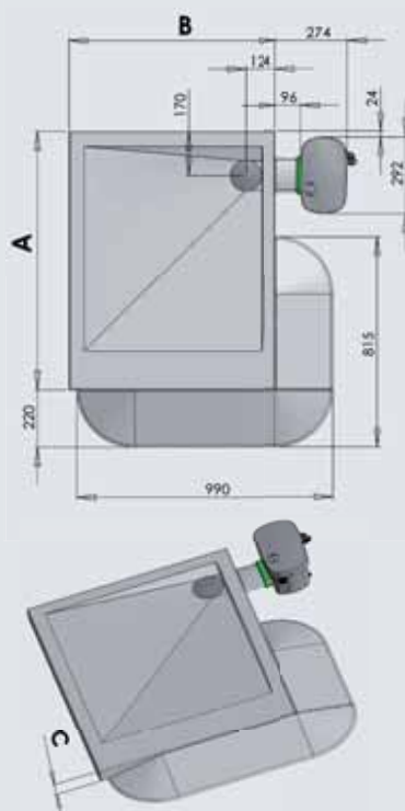
Traymatic Extern finns i 3 storlekar A×B×C: 1000×800×50 mm A×B×C: 900×900×50 mm A×B×C: 1200×800×50 mm
