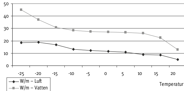
W/m Effektuttag vid olika temperaturer och omgivelningar
