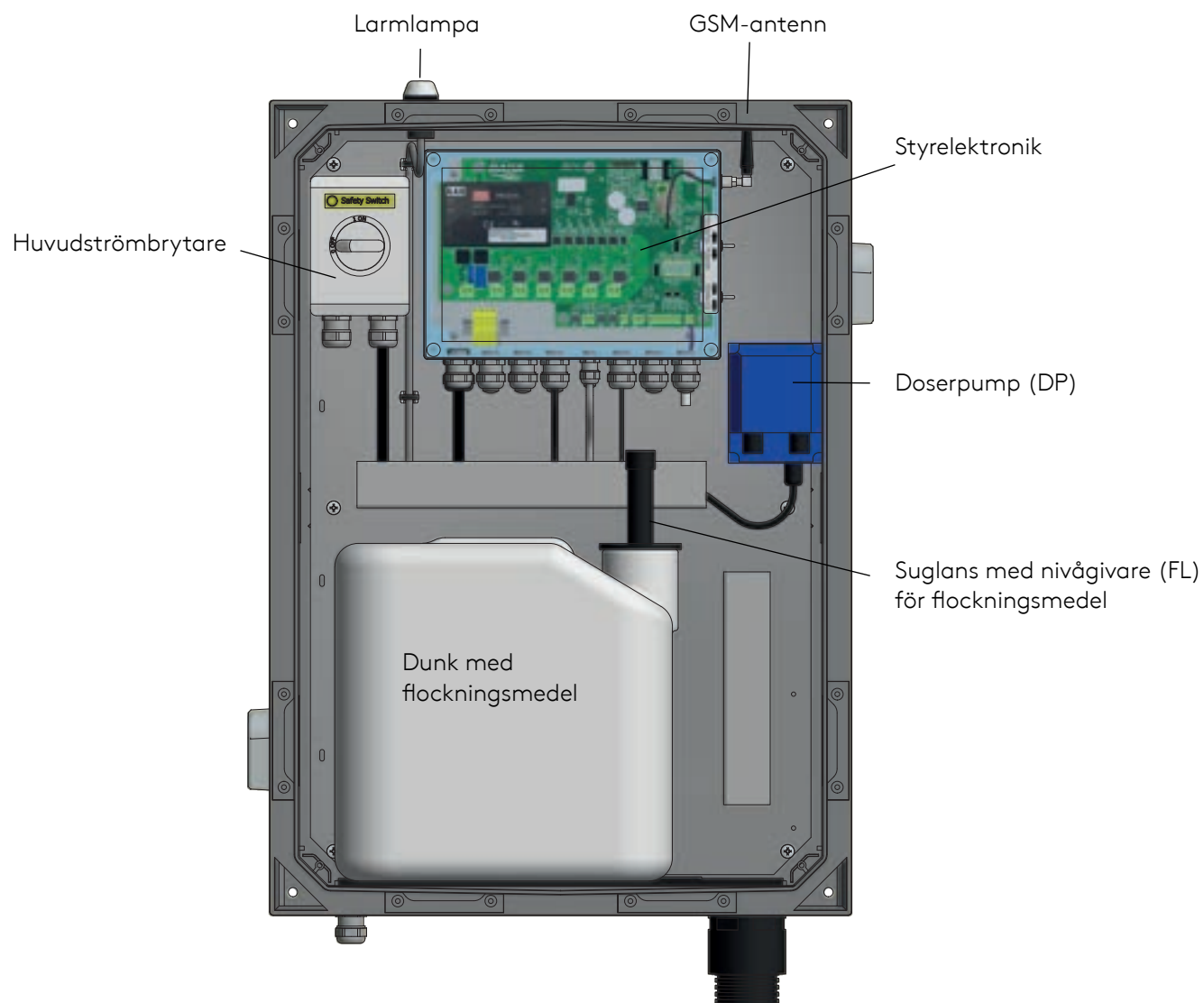
Figur 2. Översikt Automatiskåp
