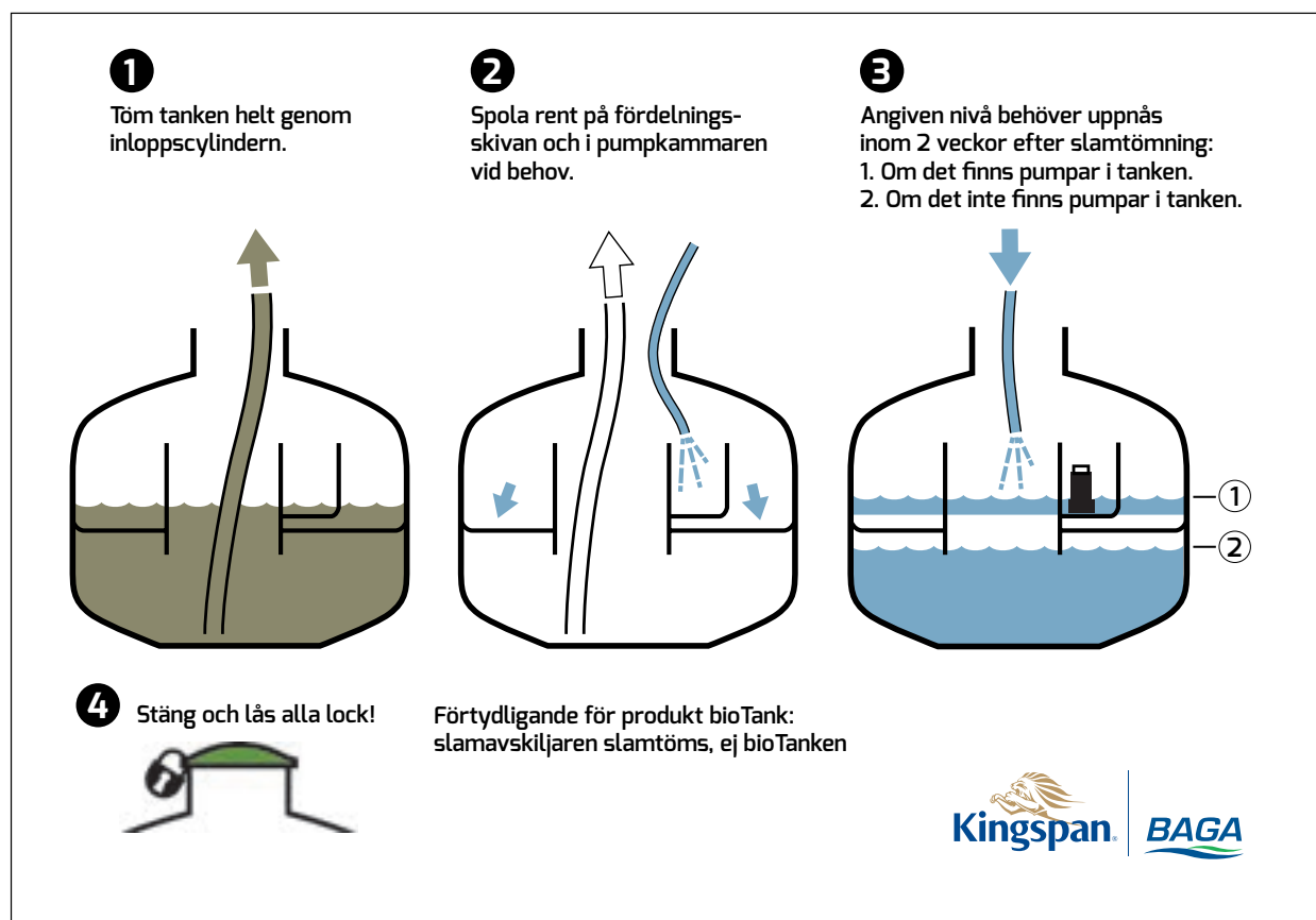
Figur 6. Slamtömningsinstruktion
